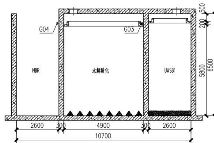
6-6剖面图
