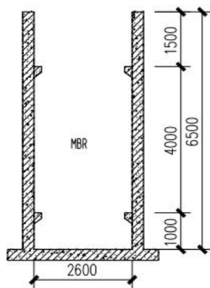
3-3剖面图
