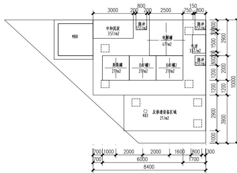
二楼设备荷载平面布置图
