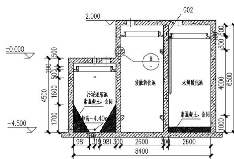
2-2 剖面图
