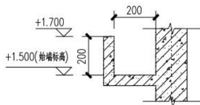
A- 出水堰大样图
