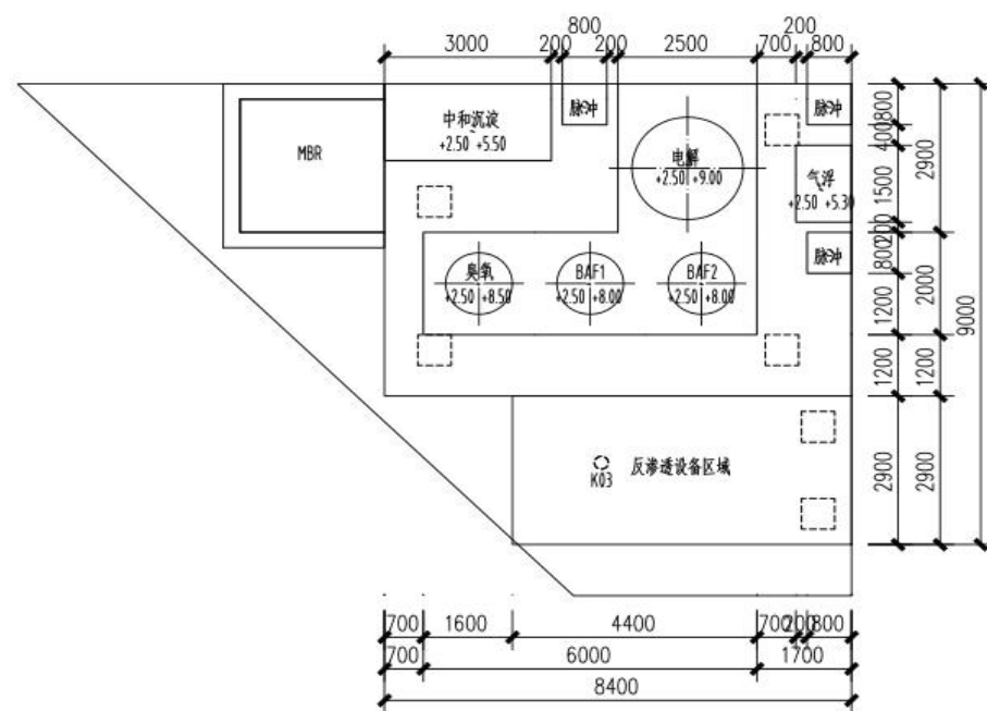
二楼平面布置图 (+2.500)
