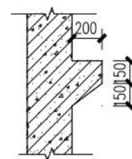
B- 牛腿大样图
