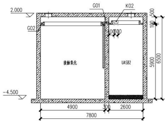
5-5剖面图
