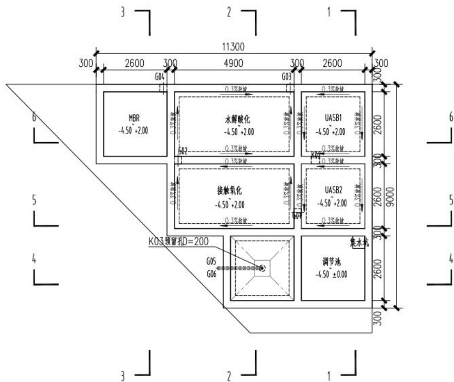
地下组合池平面布置图 (±0.000)
