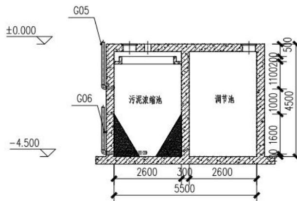
4-4剖面图
