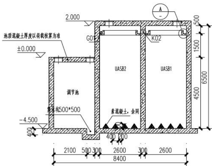
1-1 剖面图
