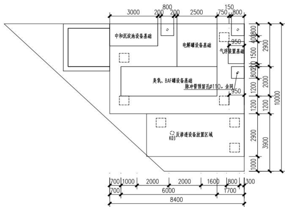
二楼设备基础平面布置图
