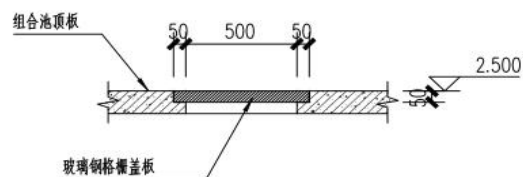
K01检修孔大样图
